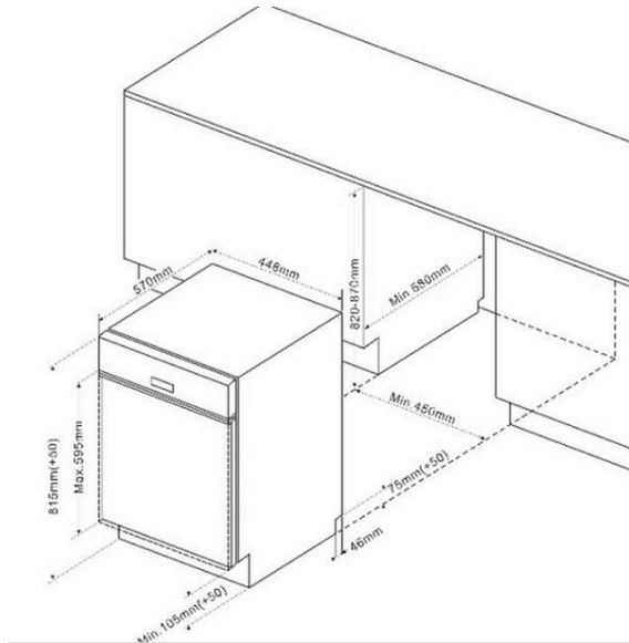
VS1010J_schéma encastrement.JPG
